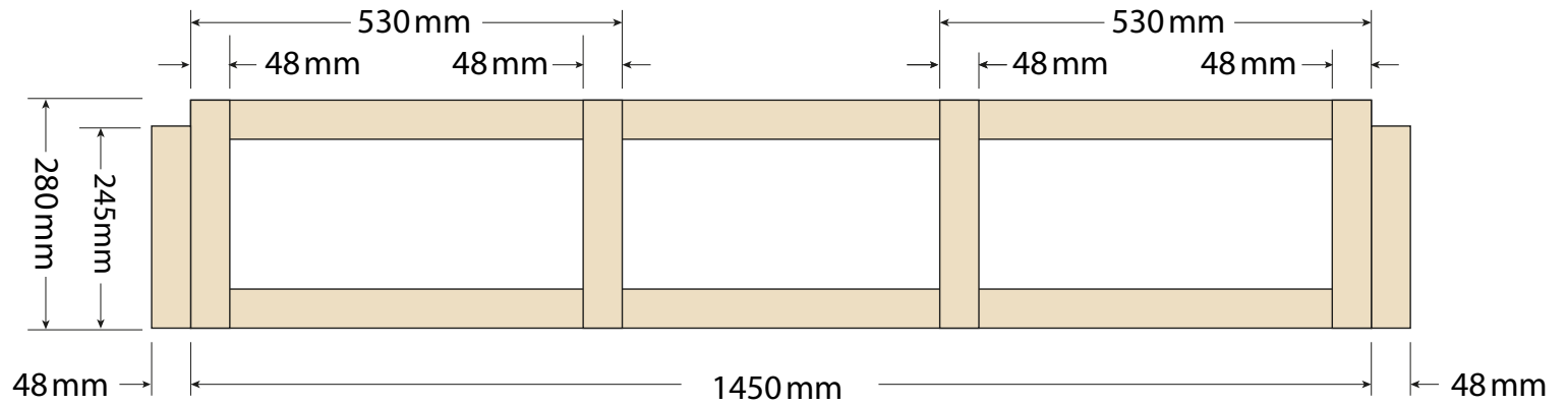
2. Table Frame
